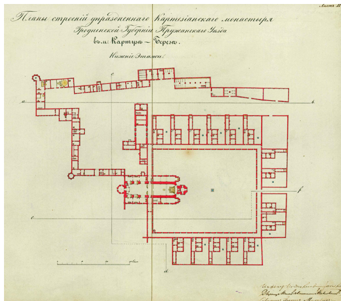
Il. 7. Kartuzja w Berezie, rzut kościoła i klasztoru, 1837. Moskwa, RGVA, 394-17-1592
