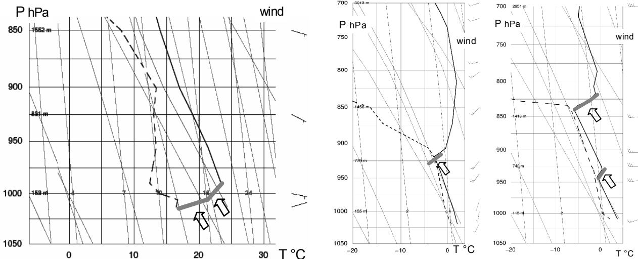
7 pav. 2004 08 04 00 GL aerolinė diagrama, sudaryta pagal Visbio (Švedija) radiozondavimo duomenis (a); 2004 12 02 00 GL aerolinės diagramos, sudarytos remiantis Lebos (Lenkija) ir Visbio (Švedija) stočių radiozondavimo duomenimis (b). Ištininės linijos žymi temperatūros, o punktyrinė – rasos taško temperatūros kreives. Pastorintos linijos ir rodyklės nurodo temperatūros inversijas
