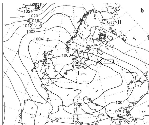
6 pav. 2004 05 04 18 GL – 05 08 12 GL 500 hPa izobarinio lygio aukštis (gpm) (a); slėgis jūros lygyje (hPa) (b); vėjo greitis (m/s) 850 hPa izobariniame lygyje (c). Izohipsės išbrėžtos kas 40 gpm, izobaros – kas 4 hPa, vėjo greitis – kas 1 m/s. Kiti specialūs ženklai kaip ir 5 pav.
